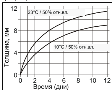
Граф.1: Скорость отвердевания Sikaflex®-291
